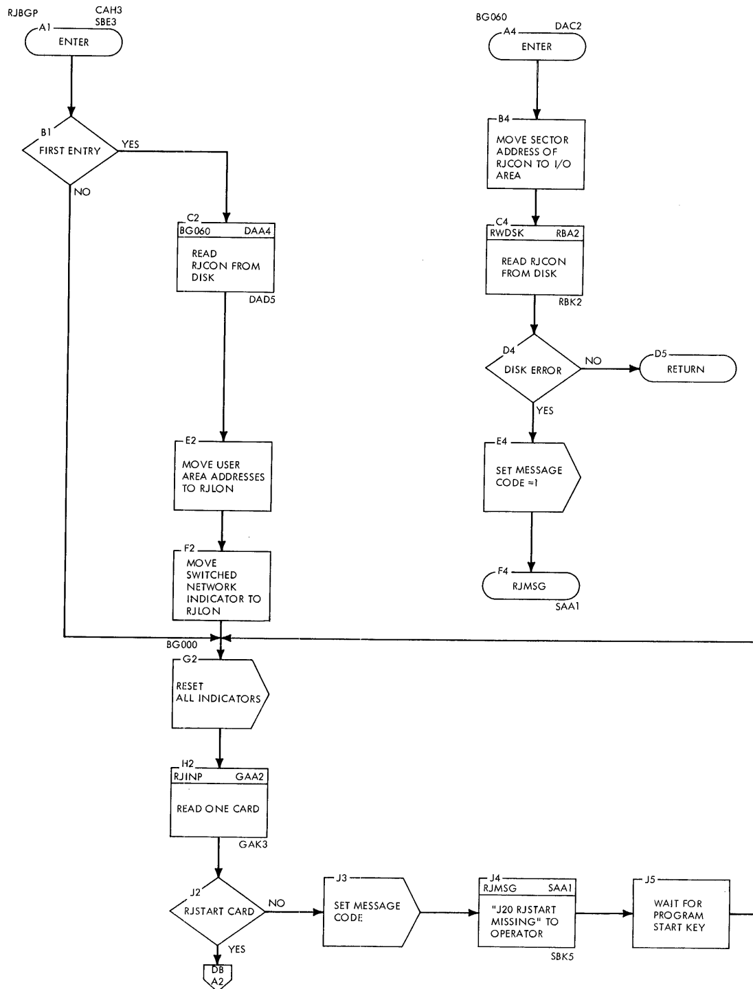
Chart DA. (RJBG) Begin Point-to-Point
